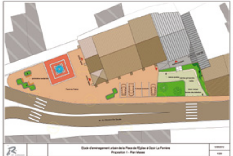
Etude d'aménagement urbain de la Place de l'église à Ozoir-la-Ferrière (plan masse)
